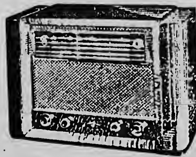
MODEL BX 718 X 6 golfbereiken 10 lampen met 13 functies Bandspreiding op: 11 - 13 16 - 20 - 25 en 30 m. band Basschakelaar in 3 standen Hoge toonregelaar en bandbreedte schakelaar PRIJS f. 330.-
